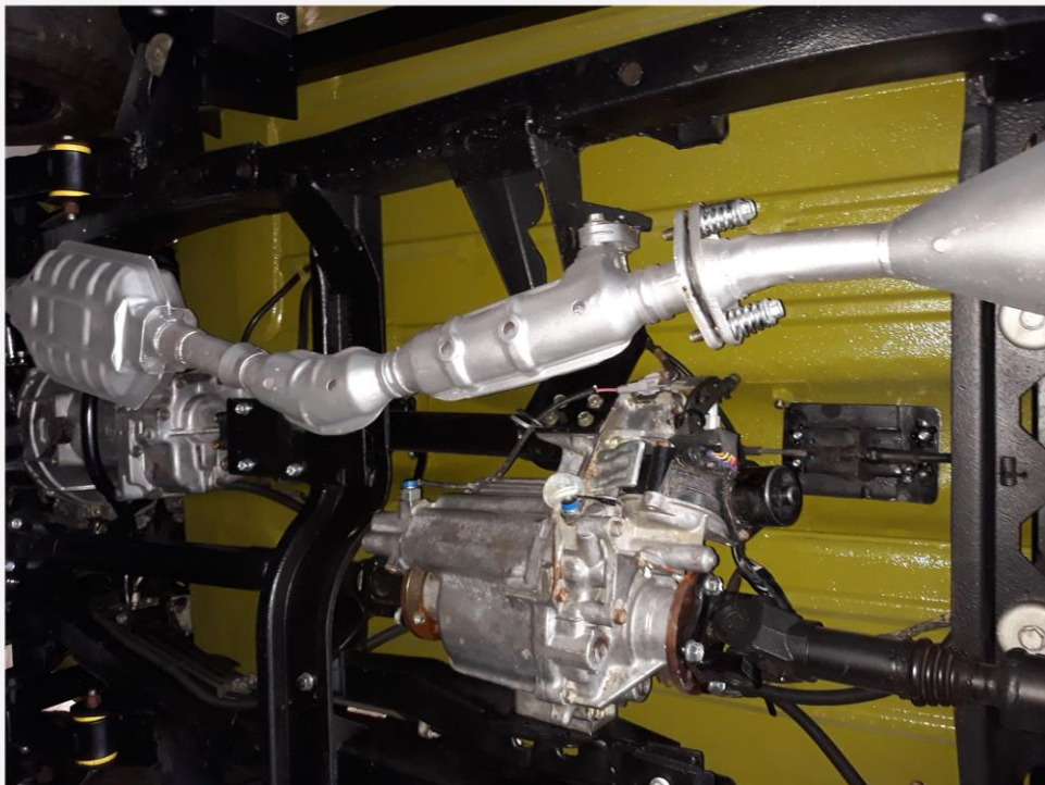
Motor und Getriebe generalüberholt, zerlegt, neu gelagert, neu abgedichtet, kürzer übersetzt. Untersetzungsgetriebe von mechanisch auf elektronisch umgebaut.
