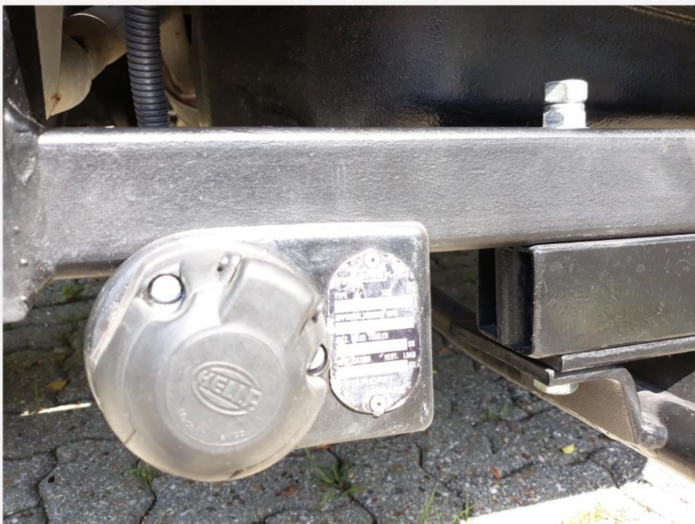
Original Suzuki Brink Anhängerkupplung mit bis zu 1100kg Anhängelast.
